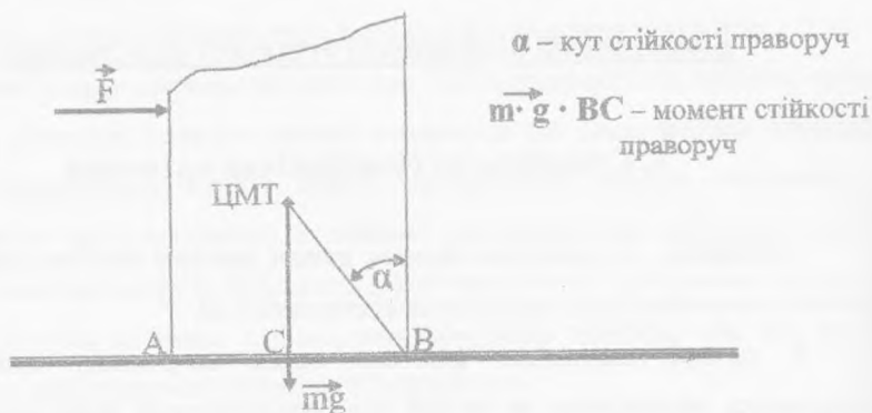
Рис. 3.1. Кут стійкості і момент стійкості тіла, що знаходиться у рівновазі.
