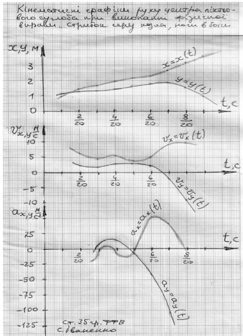
Рис. 6.1. Приклад побудови кінематичних графіків руху заданої розрахункової точки
