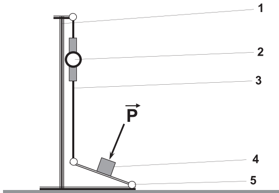
Рис. 13.3. Схема динамометра для оцінювання можливості обстежуваного точно диференціювати зусилля натиску на педаль у положенні сидячи: 1 – стійка; 2 – тяга; 3 – цифровий тензодинамометр; 4 – педаль із накладкою, що стабілізує плече прикладання зусилля; 5 – циліндричний шарнір
