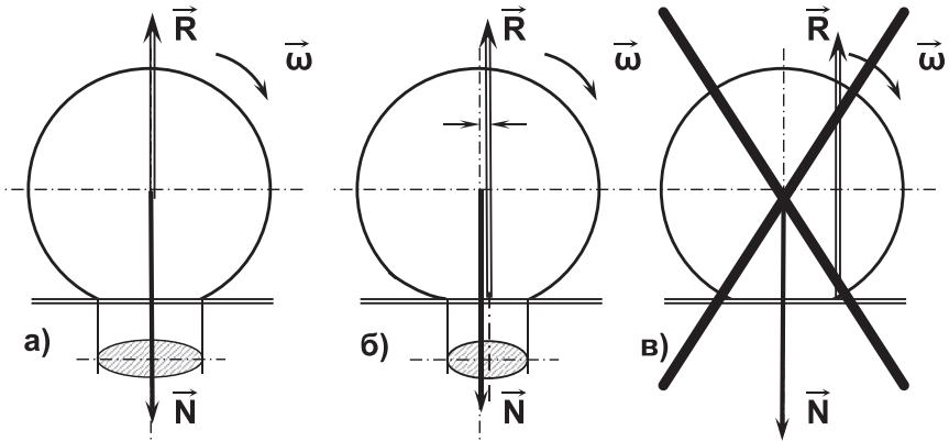
Рис. 7.1. Розрахункові схеми для визначення опору кочення колеса по горизонтальній поверхні: а) у нерухомому стані; б) під час кочення колеса; в) хибна розрахункова схема, що часто трапляється у літературі
