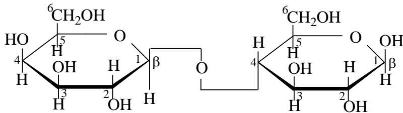
\beta -D-галактопіранозил--(1→4)- \beta -D-глюкопіраноза
