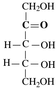
D-рибулоза
