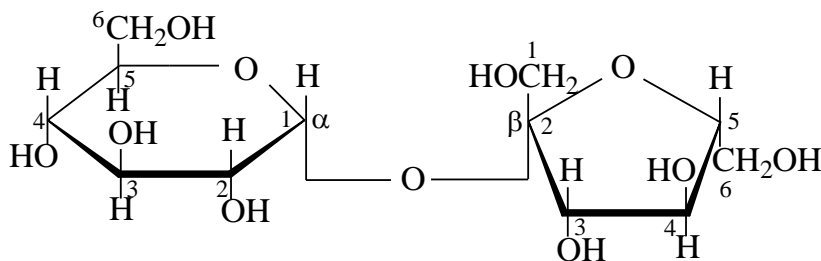
\beta -D-фруктофуранозил-(2 \rightarrow 1)- \alpha -D-глюкопіранозил
