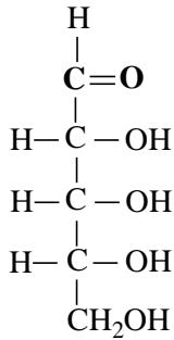
D-рибоза
