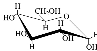
\alpha -D-глюкопіраноза
