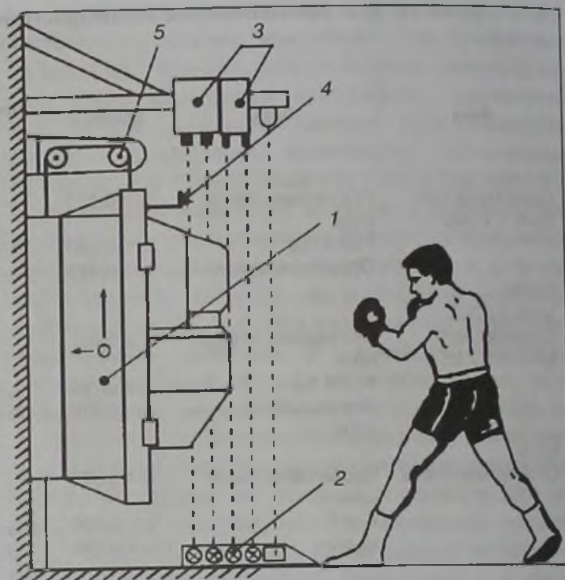
Рис. 16.11. Диагностический комплекс для оценки эффективности ударов в боксе: 1 — трехмерная динамометрическая платформа; 2 — лампы для измерения тени движения; 3 — приемное устройство для измерения тени движения; 4 — сигнальная лампа для измерения времени реакции «старт»; 5 — система, регулирующая высоту размещения платформы (Berger, 1994)
