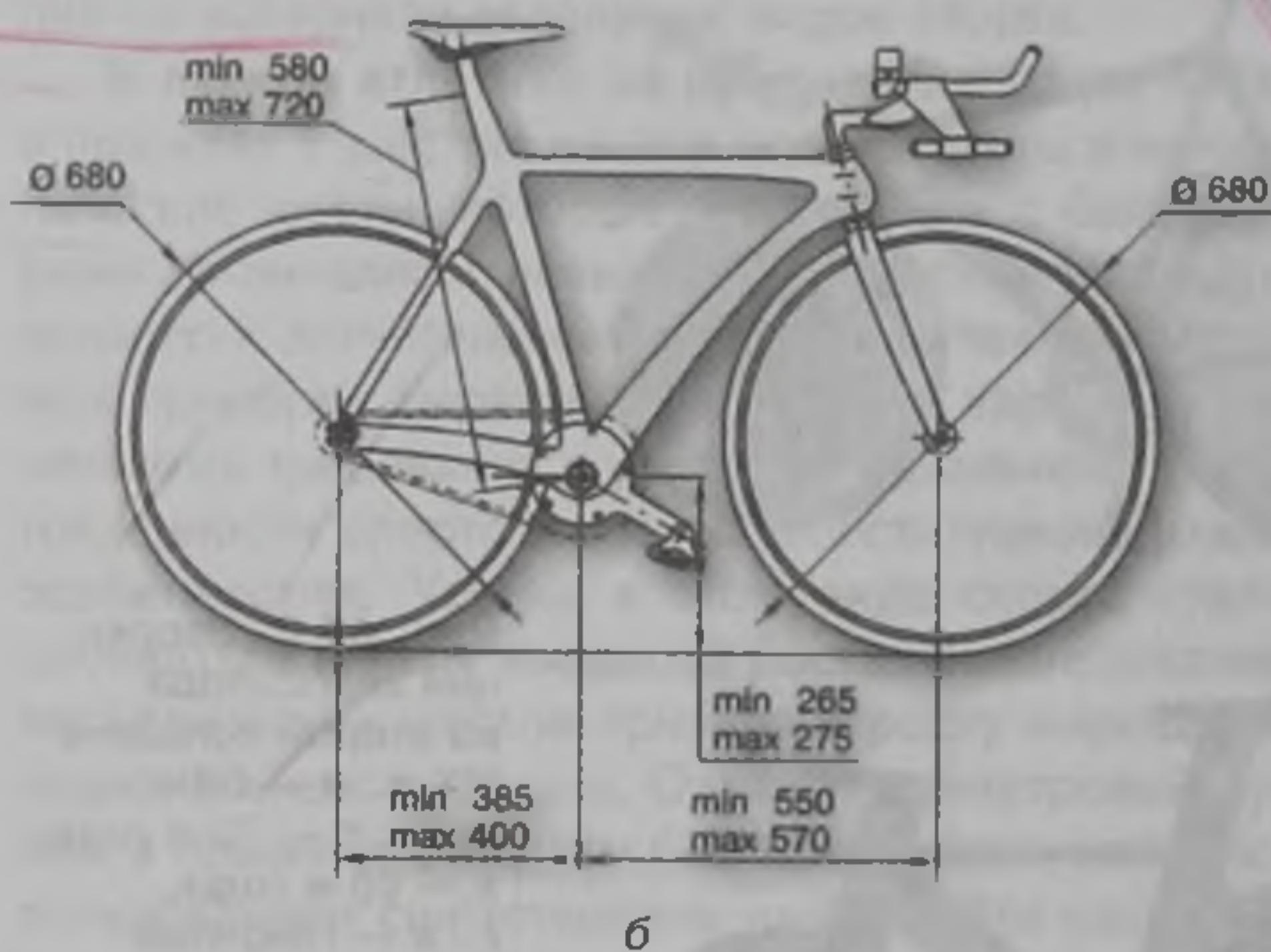
Рис. 42.4. Конструкции трековых и шоссейных велосипедов: а — велосипед трековый для спринта, б — велосипед трековый для гонок на время, в — велосипед шоссейный для гонок на время, г — на треке — чемпион мира Александр Симоненко
