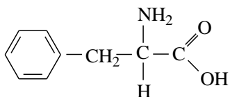
Фенілаланін
