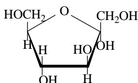
\alpha -D-фруктофураноза
