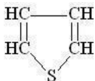
тиофен
