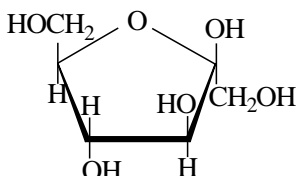
\beta -D-фруктофураноза
