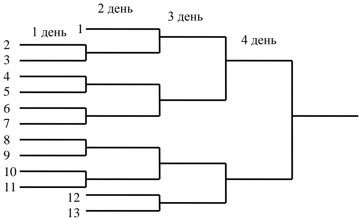
Рис. 3. Порядок зустрічей на 13 команд
