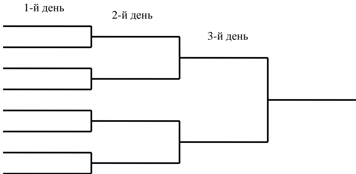
Рис. 1. Порядок зустрічей на вісім команд
