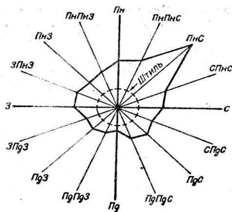
Рис. 10. Роза вітрів
