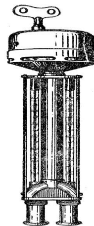
Рис. 7. Аспіраційний психрометр
