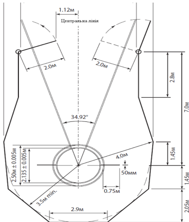
Мал. 14. Схема загороджувальної сітки для метання молоту та диска
