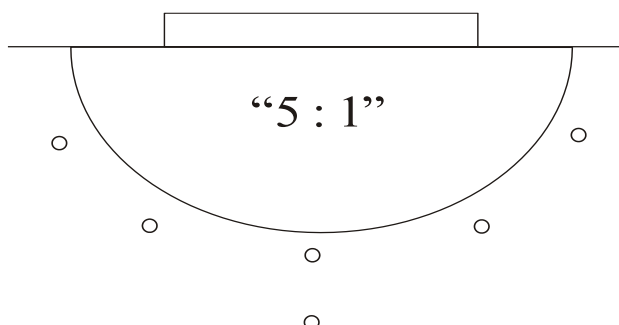
Рис. 19. Система захисту 5:1
