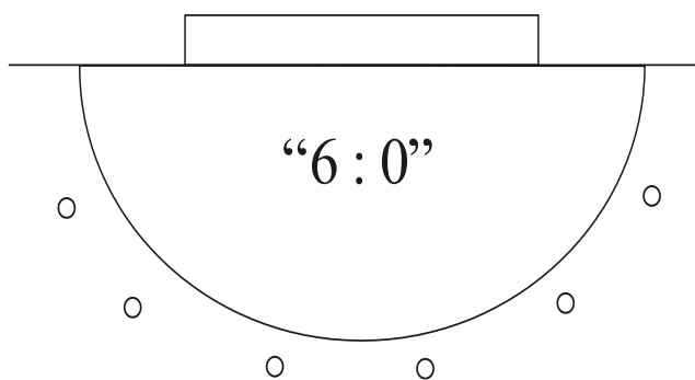
Рис. 18. Система захисту "6:0"
