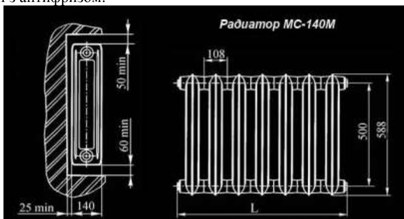
Рисунок 2 – Чавунний секційний радіатор МС-140: загальний вигляд і монтажне положення
