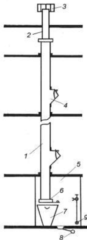
Сухий сміттепровід
