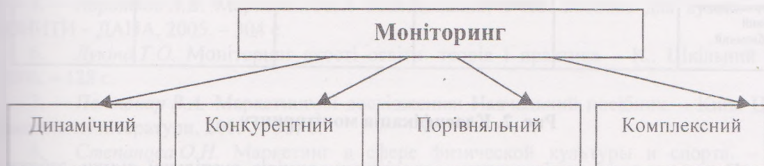
Рис. 1. Види моніторингу
