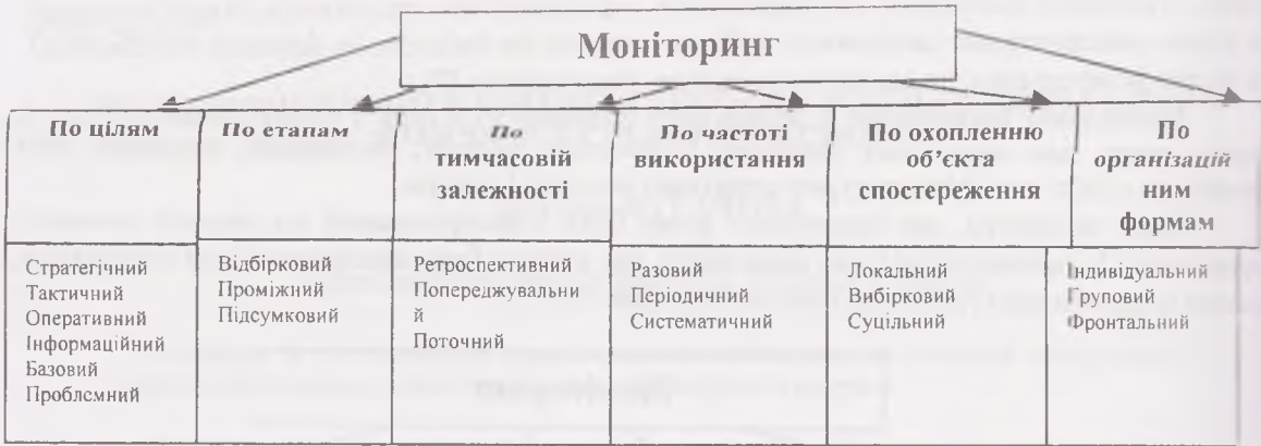
Рис. 2. Класифікація моніторингу
