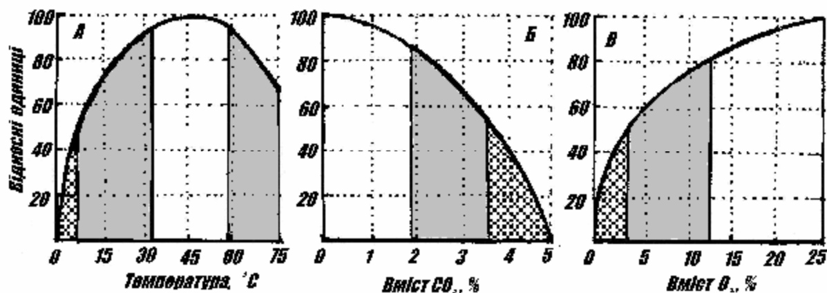
Рис. 2. Вплив температури (А), вмісту CO 2 (Б) та кисню (В) на рухливість мікроорганізмів
